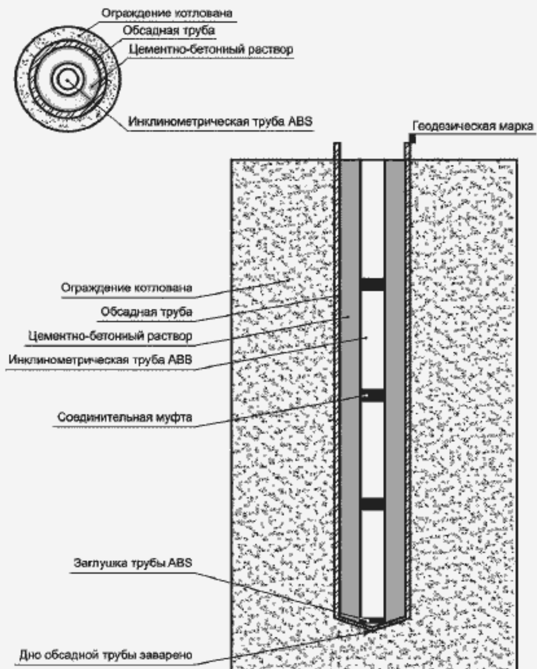
Рисунок Д.1 — Схема инклинометрической наблюдательной скважины
